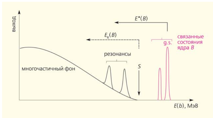
Рис.1. Схематическое представление энергетических спектров, получаемых в двухтелных реакциях. S — порог развала ядра, E^*(B) — энергия возбуждения ядра B , E_r(B) — энергия развала ядра B .
