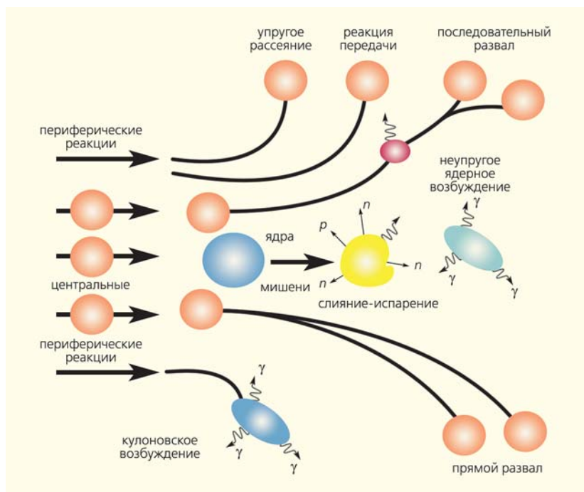
Рис.3. Различные ядерные реакции между двумя сложными ядрами для центральных и периферических столкновений. Стрелками показаны каналы «охлаждения» образующихся «горячих» ядер: прямыми — испарение протонов и нейтронов, извилистыми — вылет гамма-квантов.
