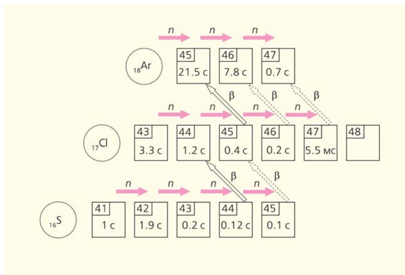
Рис.8. Карта нуклидов для нейтроноизбыточных изотопов в области S—Ar. Стрелками указаны два пути образования изотопов во Вселенной при взрыве: подхват нейтронов и β-распад. Первоначально образующиеся ядра сильно перегружены нейтронами, поэтому в результате последовательных β-распадов они начинают превращаться в более стабильные ядра, т.е. в ядра, расположенные ближе к дорожке β-стабильности. Реакции подхвата нейтронов останавливаются на так называемых «поворотных» ядрах, в данном случае это ^{44}\text{S} и ^{45}\text{Cl} .
